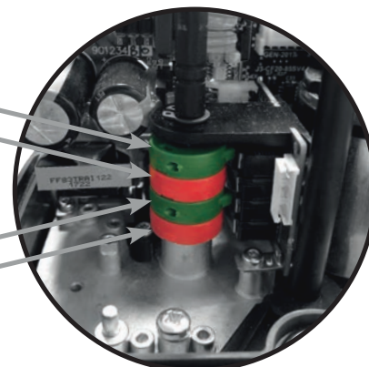
Einstellwerkzeug eingesteckt
