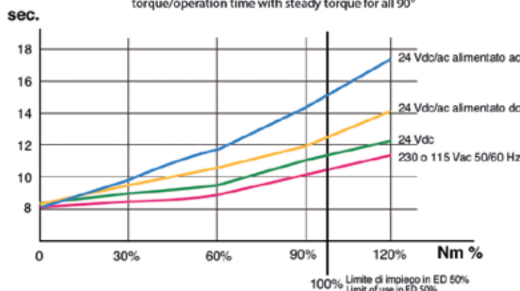
Fig.1 andamento coppia/tempo di manovra a coppia costante per tutti i 90° di lavoro torque/operation time with steady torque for all 90°
